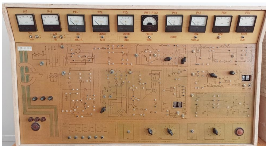
Зертханалық стендтер: «Электротехника»
