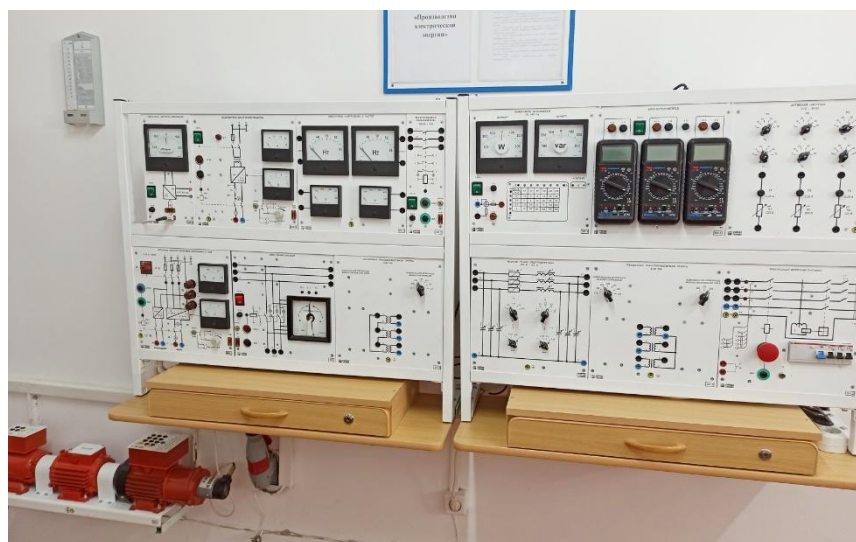
«Темір жолдарды электрмен жабдықтау»
